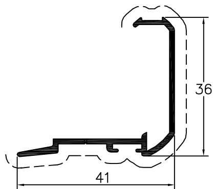
Perfil de Encaixe 90300
