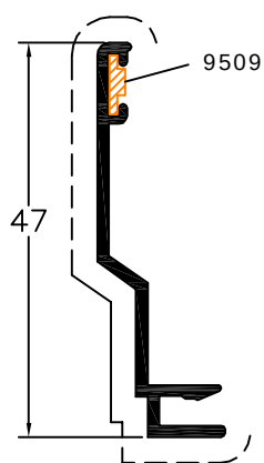
Pingadeira 80003
