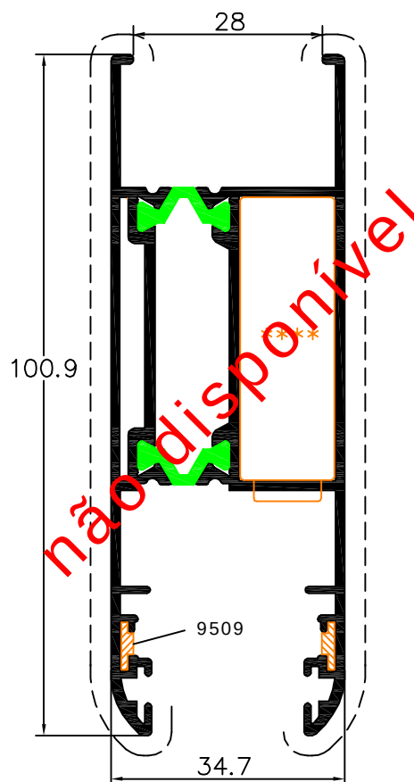
Aro Movél 90201
