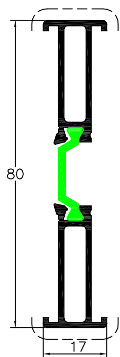
Perfil Ligação 91010
