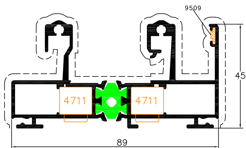
Aro Fixo 90101
