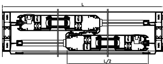
Janela de 2 Folhas
