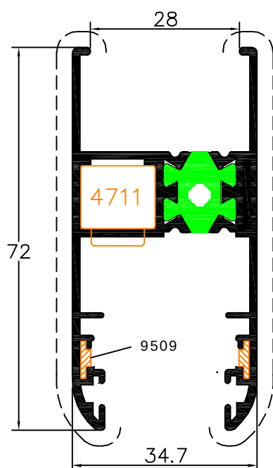
Aro Movél 90200
