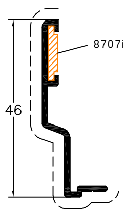
Pingadeira 80002
