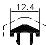
Guia Rolamento 80050
