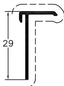
Perfil de Remate AL.1837
