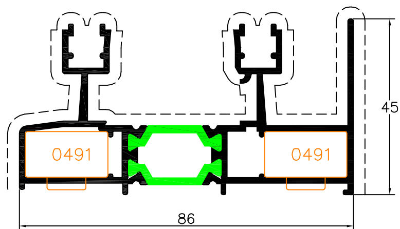
Aro Fixo 90100
