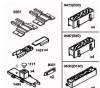
Kit para 2 Folhas A5095.D150 A5095.S60 A5095.S30
