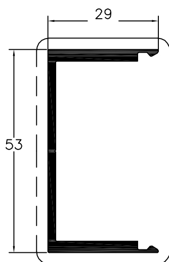
Perfil de Reforço 80030
