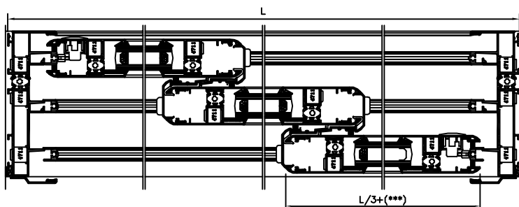
Janela de 3 Folhas
