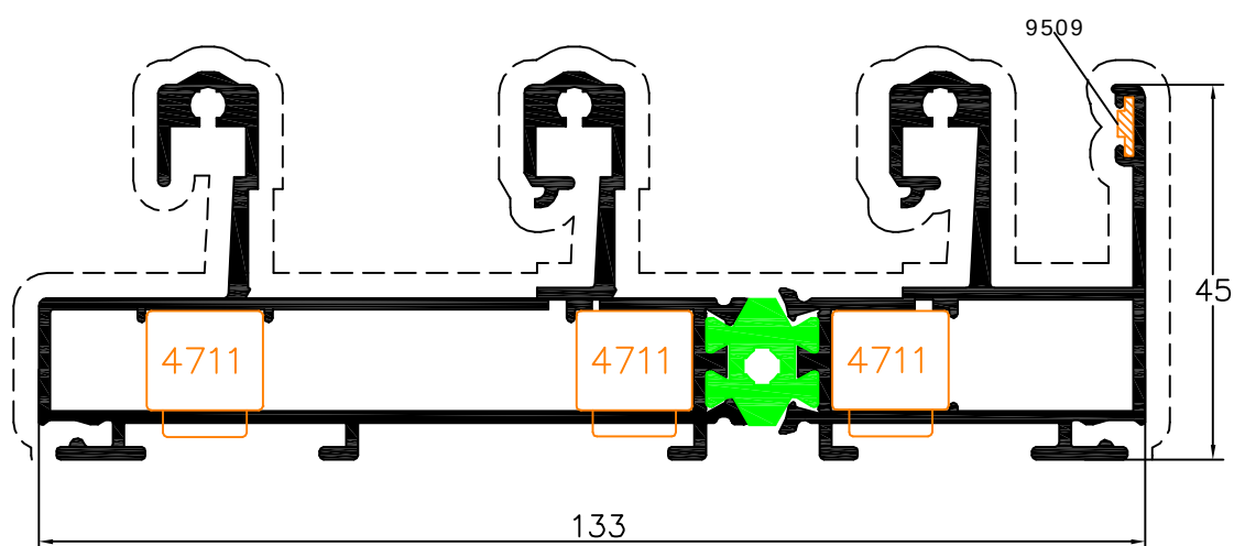
Aro Fixo Tri-Rail 90103
